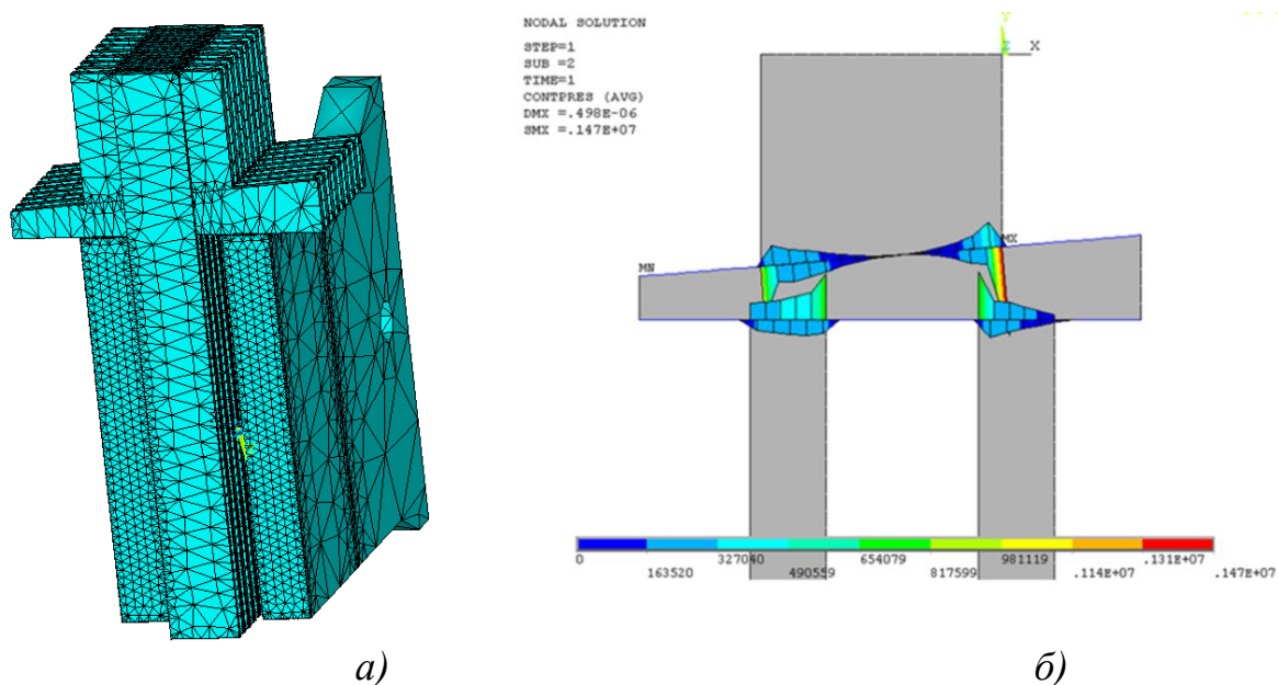
Рис. 2. Конечно-элементная модель (а) и эпюра контактных давлений (б)
