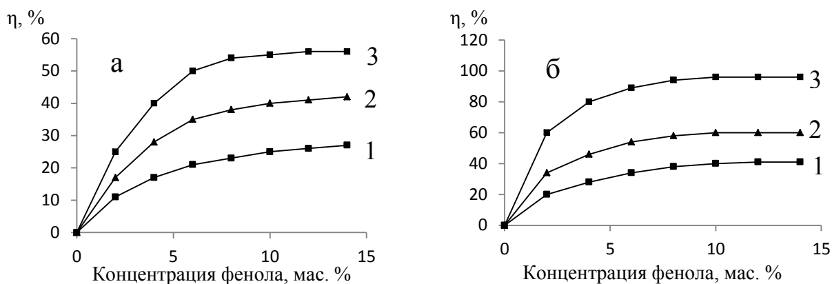
Рис. 3. Влияние концентрации фенола на степень его извлечения исходным (а) и модифицированным (б) древесным сорбентом при температурах: 1 – 293 К; 2 – 313 К; 3 – 333 К (фракционный состав сорбента 0,5... 5,0 мм, \tau = 15 мин)
